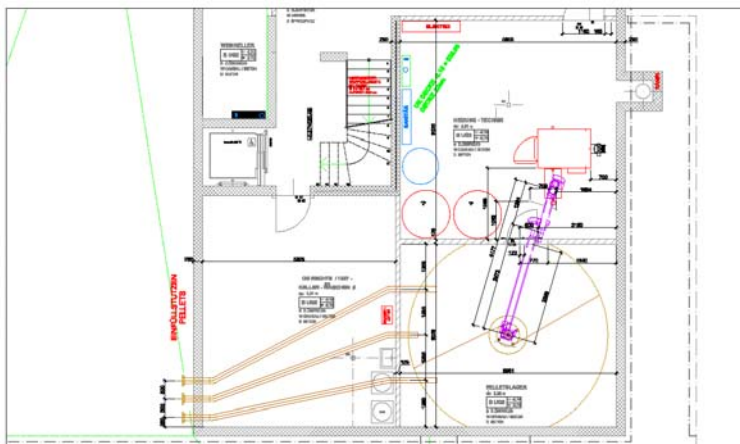
Port, Jardin Bellevue Typ: SL-T 150 kW RIBEN Grundriss 1
